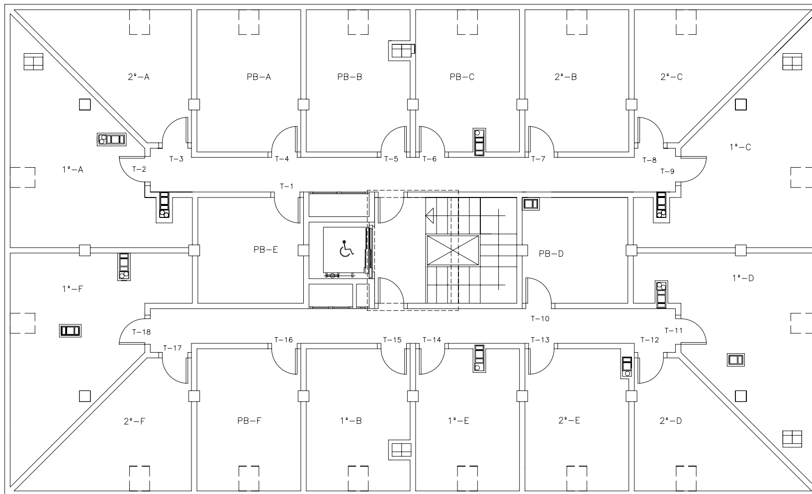
PLANTA BAJOCUBIERTA, TRASTEROS BLOQUES 1 Y 2
